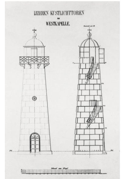
Bouwtekening uit 1875.
